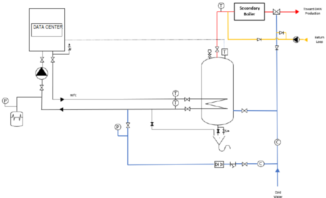
Διάγραμμα εγκατάστασης πράσινου κέντρου δεδομένων σε κλειστό βρόχο
