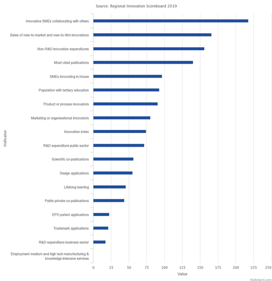
Γράφημα 9: Το προφίλ της Δυτικής Μακεδονίας – 2019, Σύγκριση με ΕΕ - 2011 EL53 – Dytiki Makedonia Profile in 2019 compared with the EU in 2011
