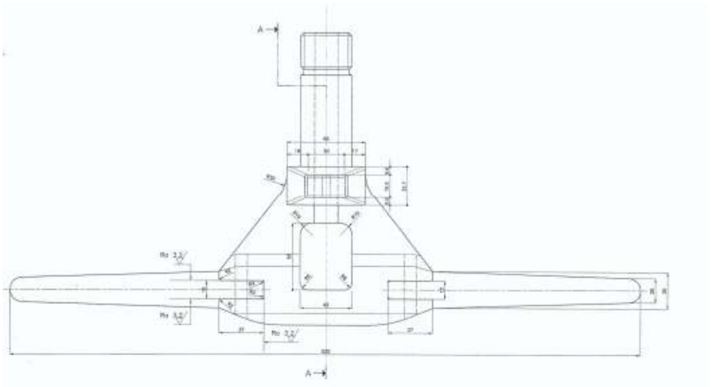
ΣΧΕΔΙΟ 1: Κάτοψη από το υπό προμήθεια σταθερό σώμα κλέμας (ενδεικτικό σχέδιο)
