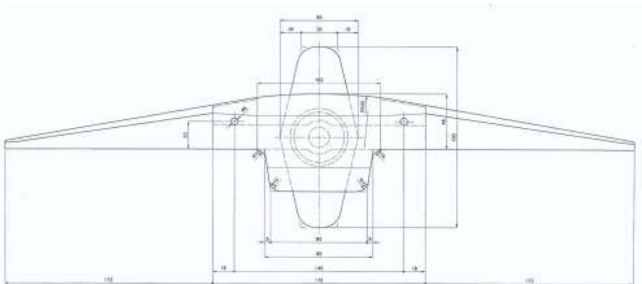
ΣΧΕΔΙΟ 2: Πλάγια όψη από το υπό προμήθεια σταθερό σώμα κλέμας (ενδεικτικό σχέδιο)
